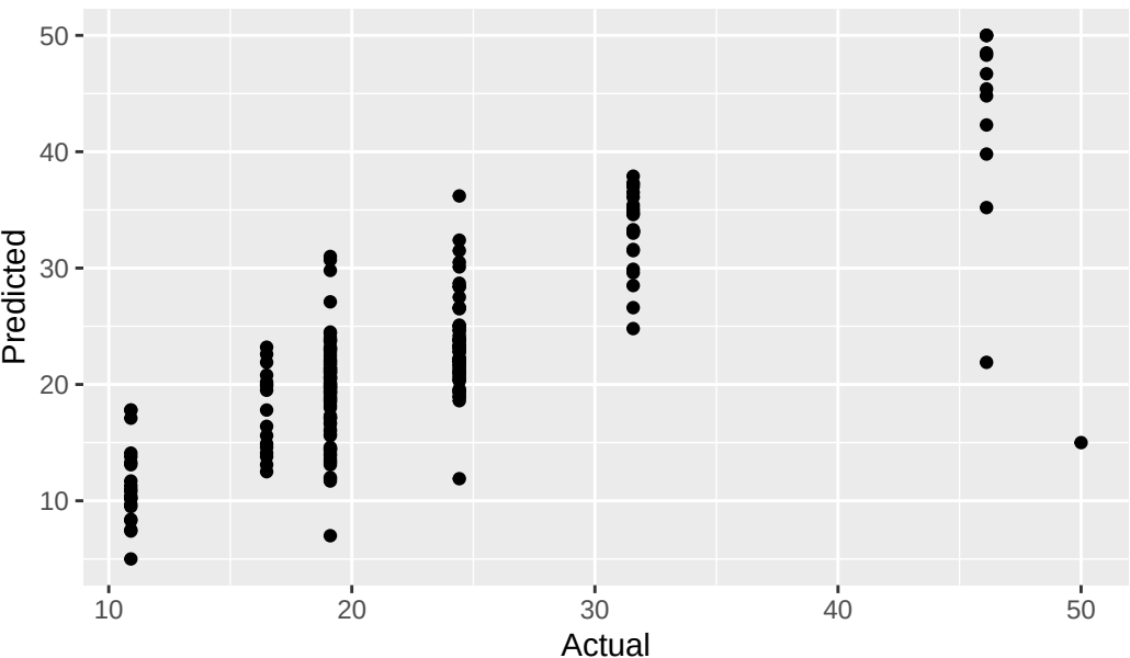
Linear predicted vs actual
